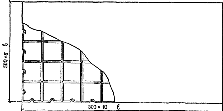
ГИБКАЯ ЖЕЛЕЗОБЕТОННАЯ ПЛИТА ПГ-10; ПГ-12; ПГ-15
