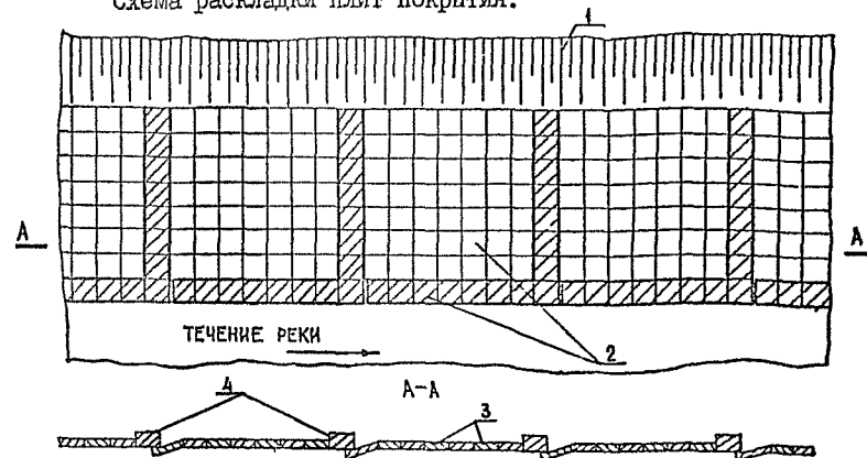
1- БЕРЕГОВАЯ СТОРОНА; 2- КАРТЫ ПОКРЫТИЯ; 3- ЖЕЛЕЗОБЕТОННЫЕ ПЛИТЫ МАССЫ, РАВНОЙ 0,5 РАСЧЕТНОЙ; 4- ЖЕЛЕЗОБЕТОННЫЕ ПЛИТЫ РАСЧЕТНОЙ МАССЫ
