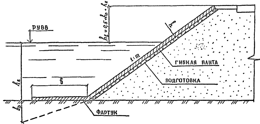
ГИБКАЯ ЖЕЛЕЗОБЕТОННАЯ ПЛИТА ПГ-10; ПГ-12; ПГ-15
