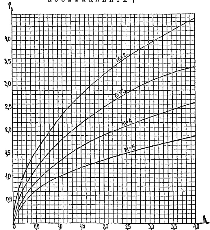
ГРАФИК ДЛЯ ОПРЕДЕЛЕНИЯ КОЭФФИЦИЕНТА \varphi
