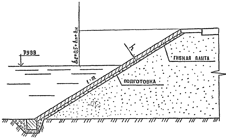
ГИБКАЯ ЖЕЛЕЗОБЕТОННАЯ ПЛИТА ПГ-5; ПГ-75
